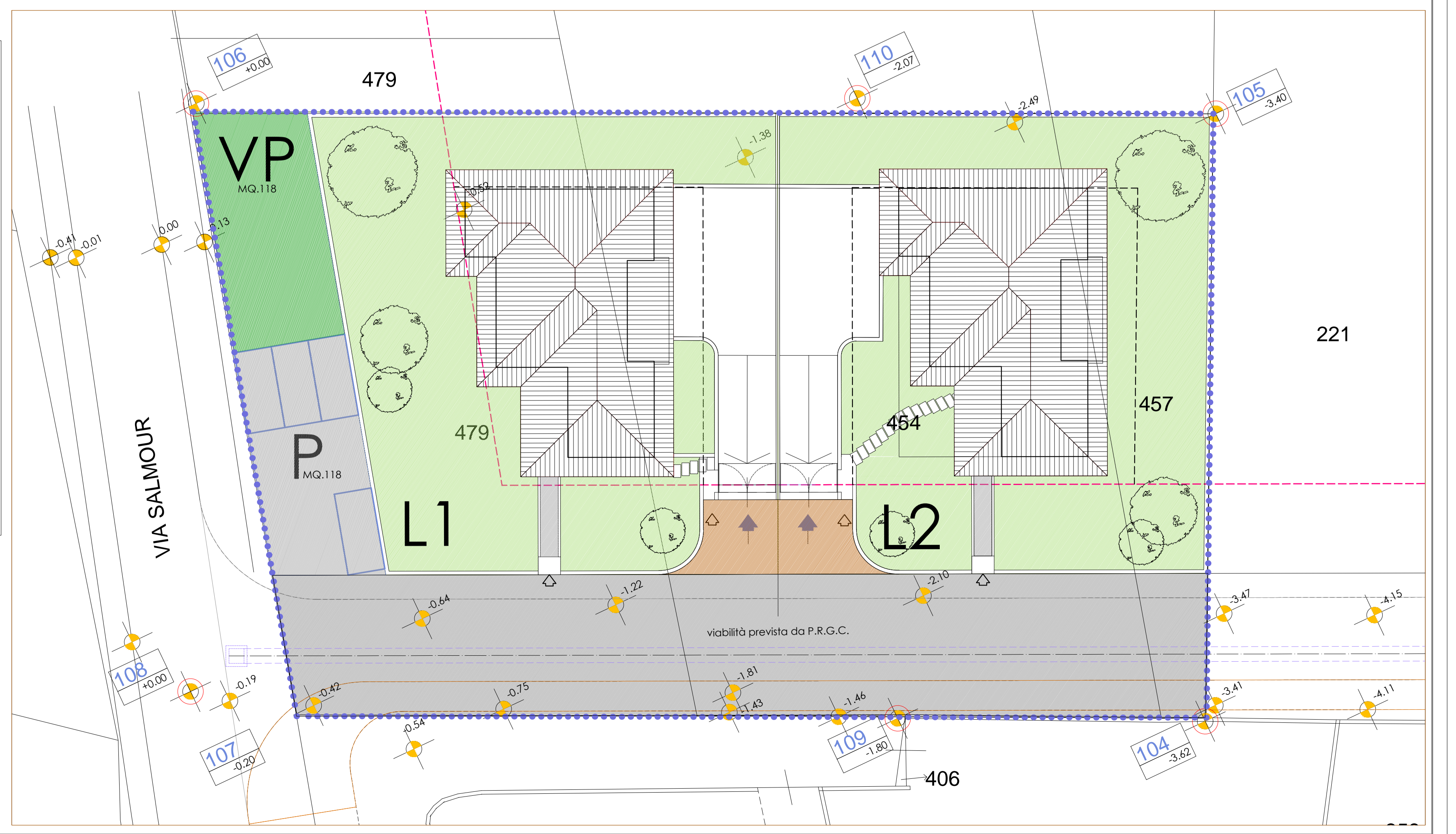
PLANIMETRIA DI PROGETTO scala 1:200
